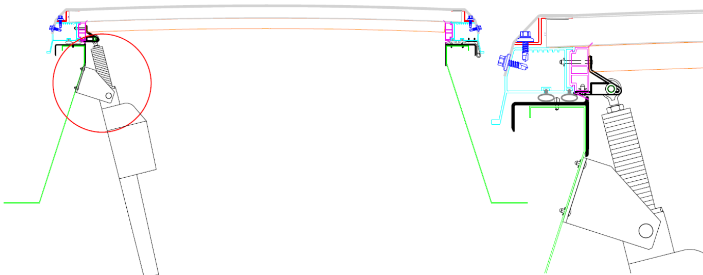
Rys. 31. Mocowanie konsoli dolnej siłownika elektrycznego do podstawy skośnej
