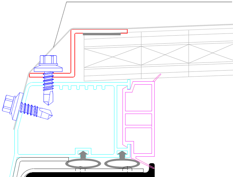
Rys. 26. Montaż taśmy aluminiowej za pomocą wkrętów samowiercących c.d.
