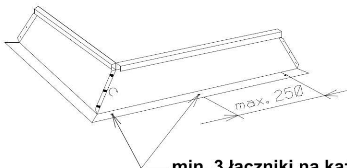
Rys. 13. Rozstaw i ilość łączników
