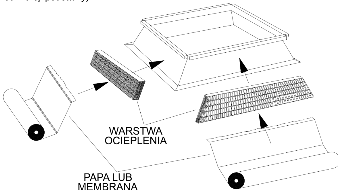
Rys. 14. Ocieplenie podstawy
