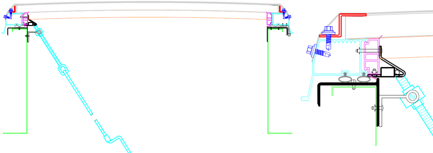
Rys. 32. Mocowanie konsoli dolnej ręcznego otwieracza śrubowego
