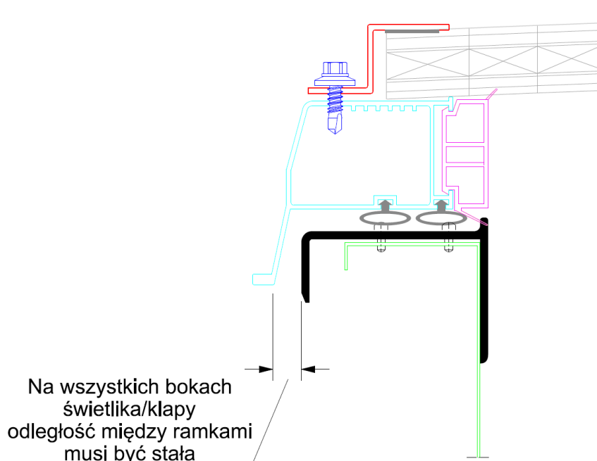
Rys. 22. Montaż zetownika zamykającego do ramki aluminiowej za pomocą śrub samowierących
