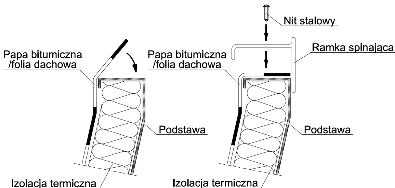
Rys. 15. Wywinięcie obróbki dachowej na górną półkę podstawy
