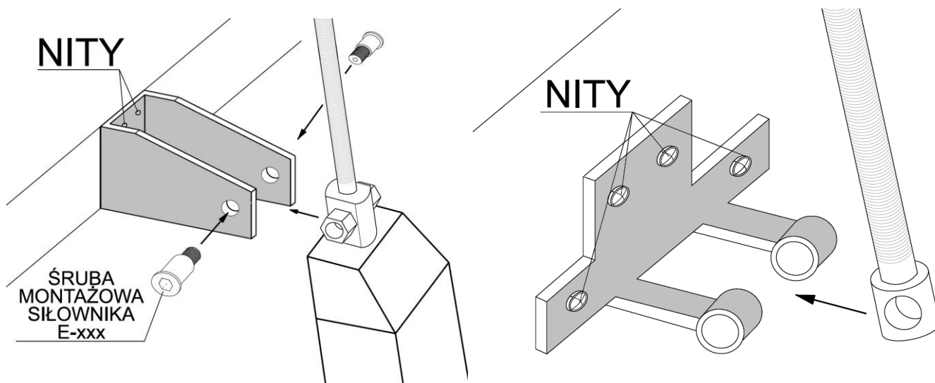
Rys. 34. Mocowanie korpusu siłownika elektrycznego / otwieracza śrubowego do konsoli dolnej
