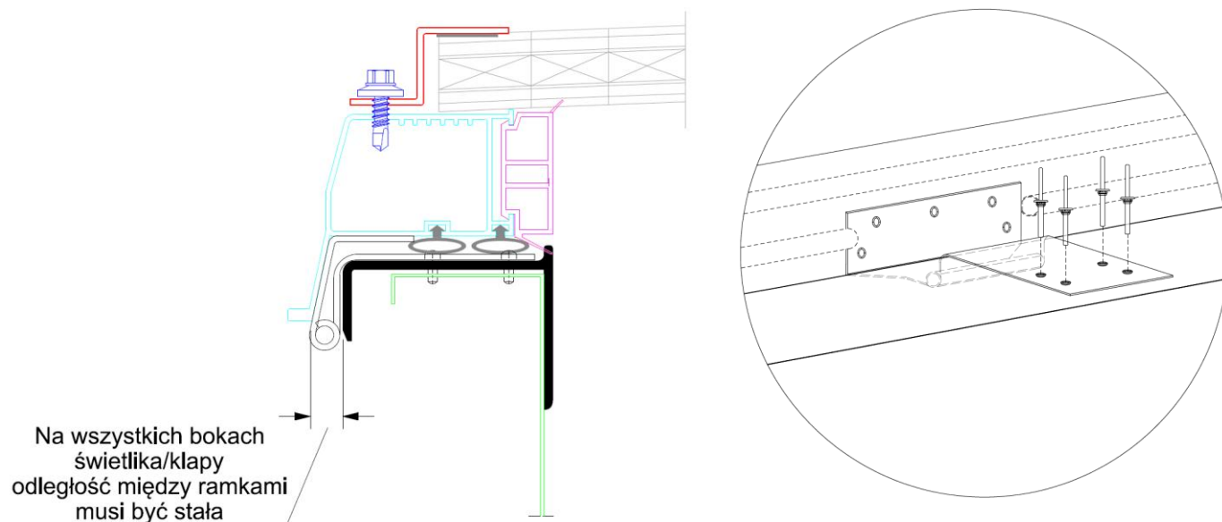
Rys. 27b. Mocowanie ramki zawiasowej c.d.
