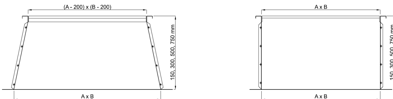
Rys. 1. Podstawa skośna i prosta z blachy stalowej ocynkowanej
