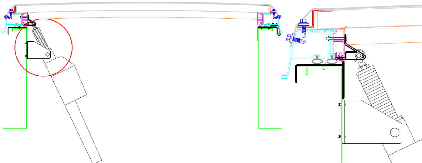
Rys. 30. Mocowanie konsoli dolnej siłownika elektrycznego do podstawy prostej
