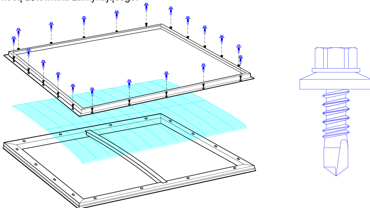
Rys. 21. Montaż płyty poliwęglanowej oraz zetownika zamykającego na ramce aluminiowej
