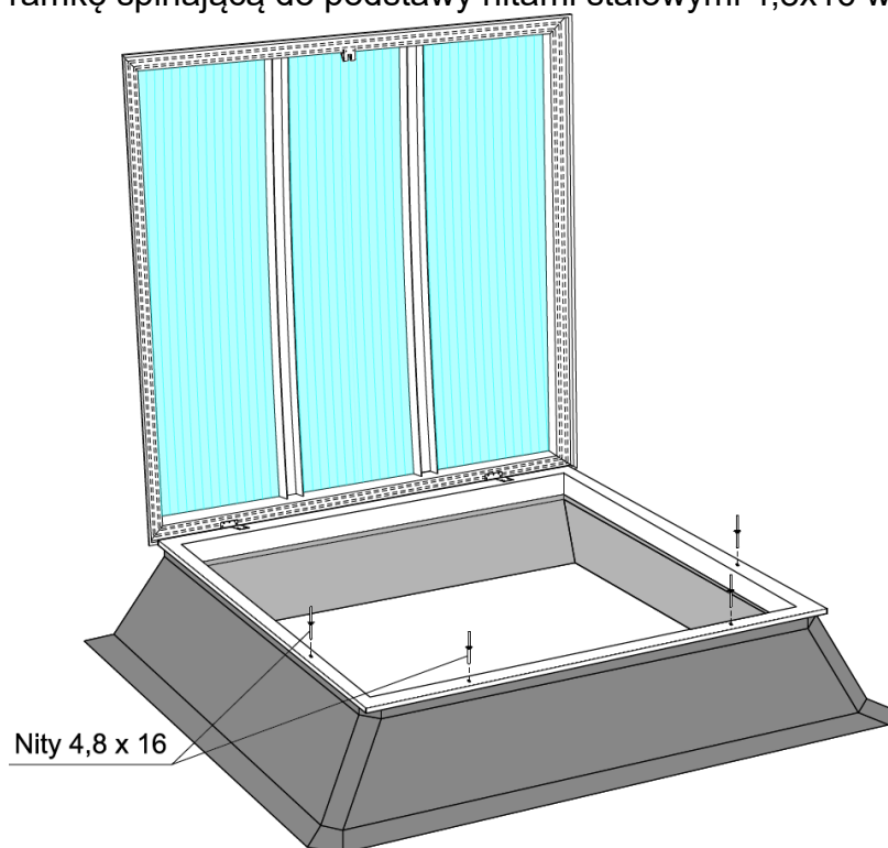
Rys. 28. Mocowanie ramki spinającej
