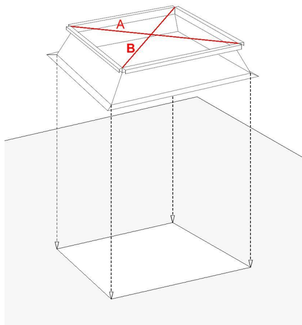
Rys. 12. Przymocowanie podstawy wylazu do konstrukcji nośnej dachu
