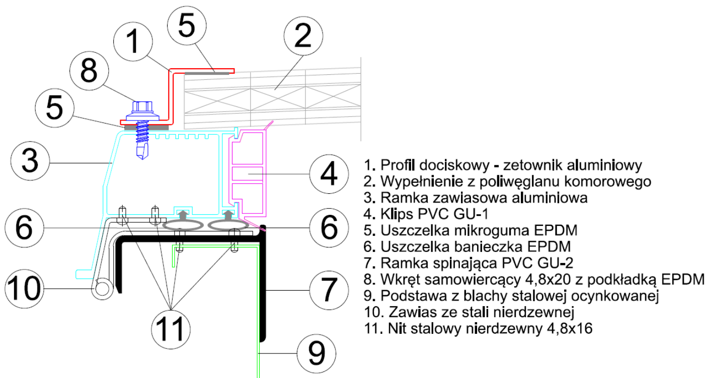
Rys. 3a. Przekrój przez konstrukcję segmentu uchylnego świetlika otwieranego, podstawa z blachy stalowej
