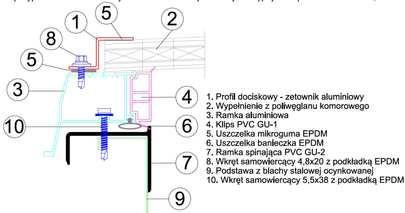
Rys. 3b. Przekrój przez konstrukcję świetlika stałego, podstawa z blachy stalowej
