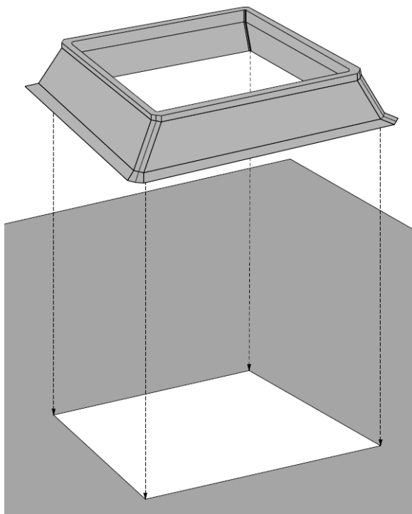
Rys. 17. Montaż podstawy z laminatu
