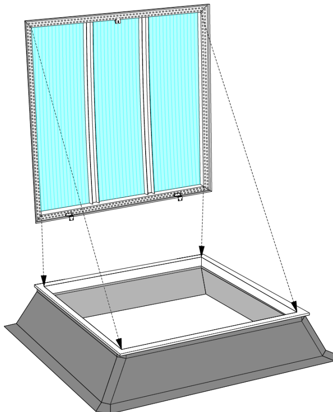
Rys. 27. Mocowanie ramki zawiasowej
