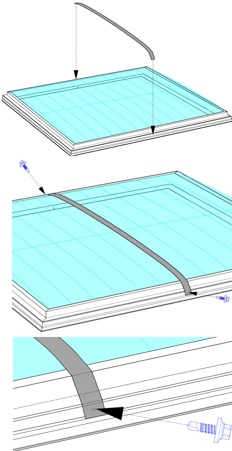
Rys. 23-25. Montaż taśmy aluminiowej za pomocą wkrętów samowiercących
