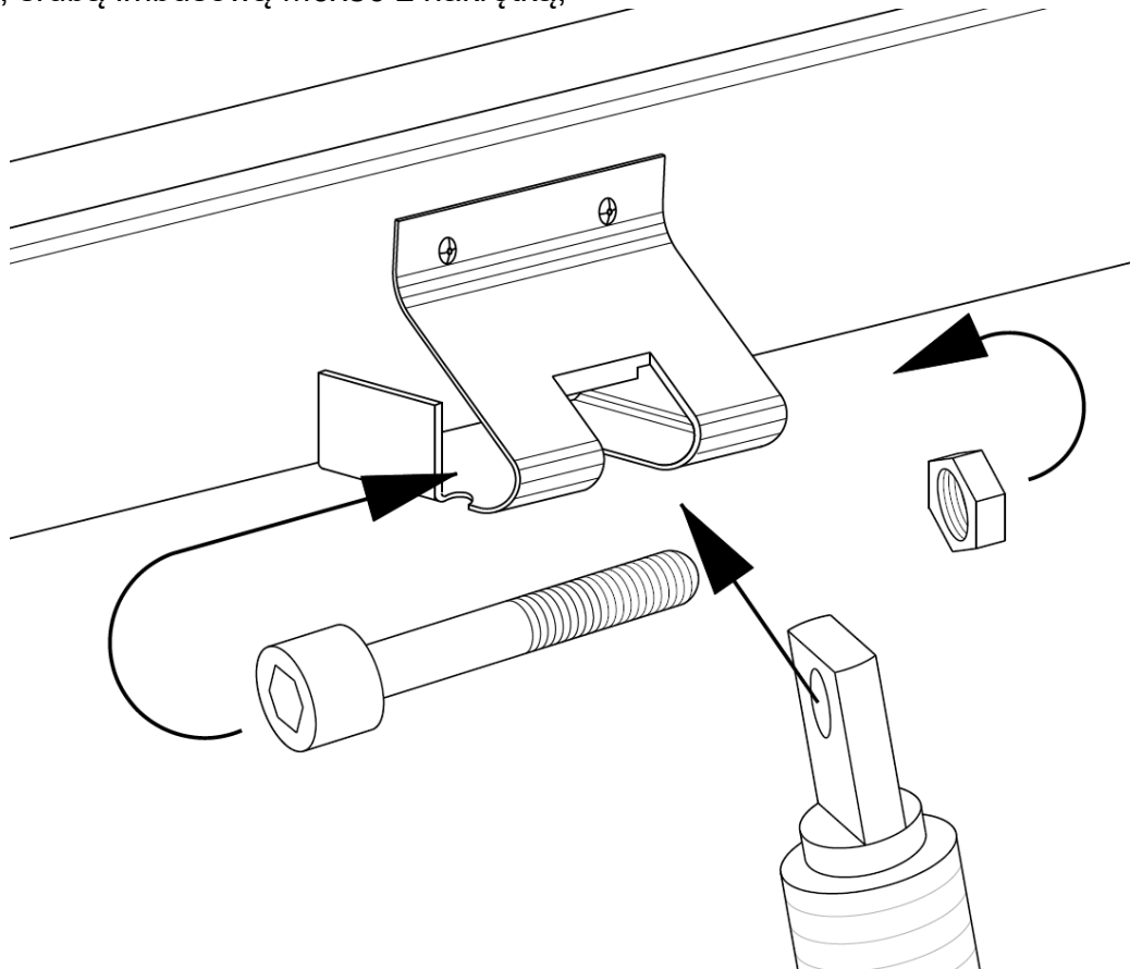
Rys. 33. Mocowanie oczka wrzeciona do konsoli górnej
